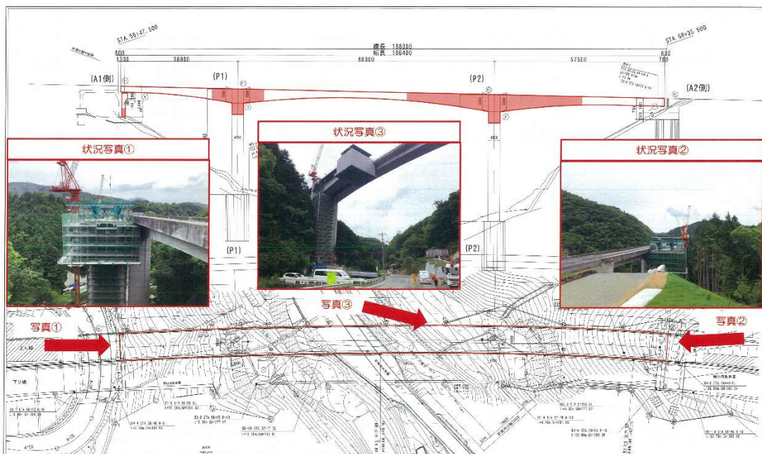
川関橋 全体一般図
