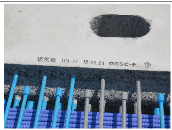
PC 版とジベル筋設置箇所
