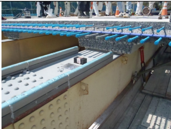
鋼桁下処理と新設 PC 床版
